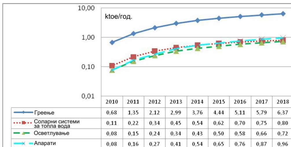
Слика 1.1.2.6. Придонес на симулираните мерки во потенцијалот за вкупни енергетски заштеди од енергетските кодекси за градежни објекти во резиденцијалниот сектор
