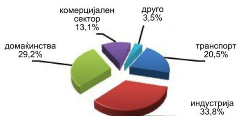
Слика 1.2. Потрошувачка на финална енергија по сектори, во 2006 година
