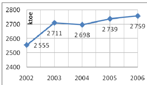
Слика 1.1. Снабдување со примарна енергија во анализираниот период
