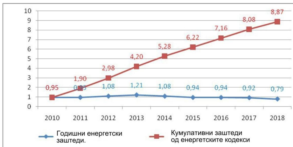
Слика 1.1.2.7. Стапка на продирање на енергетските кодекси за градежни објекти и годишни заштеди
