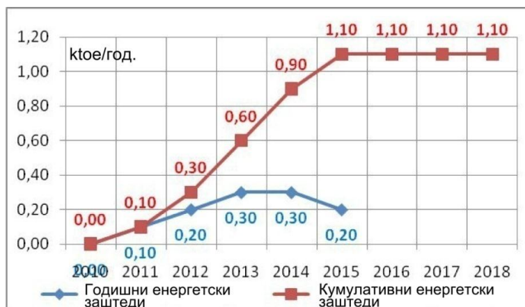
Слика 1.2.2.2. Тренд на енергетски заштеди што се должи на контролата на котли за топла вода
