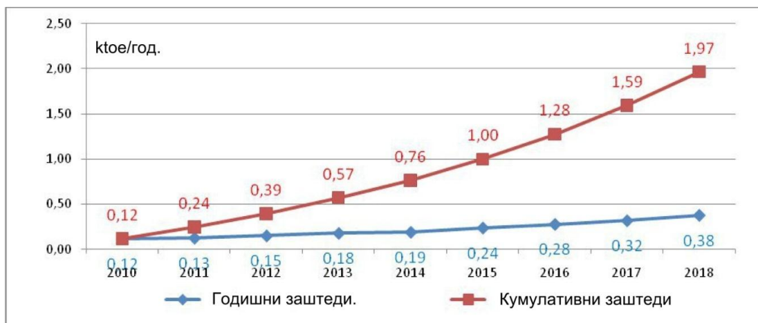
Слика 1.1.2.11. Тренд на енергетски заштеди од контролата на котли за топла вода и клима уреди
