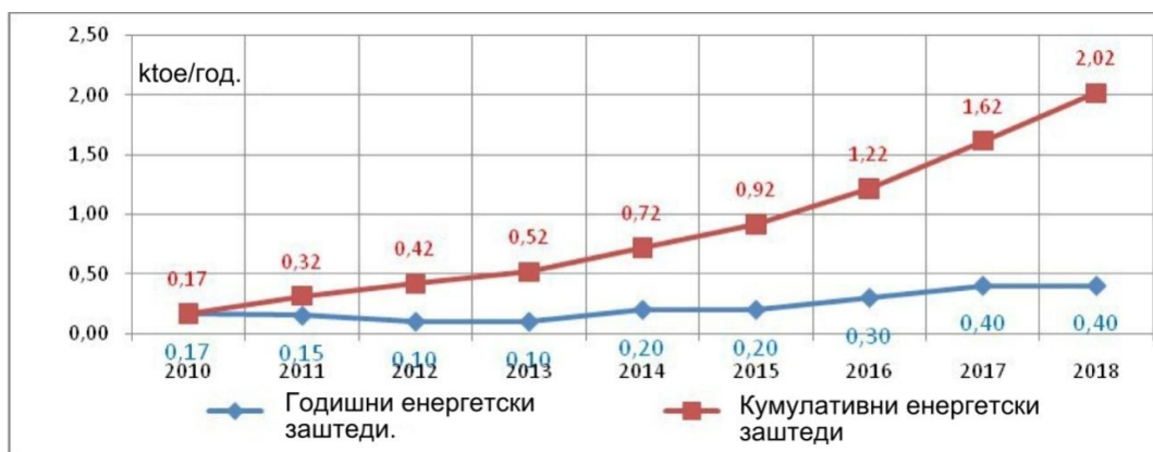
Слика 1.1.2.12. Енергетски заштеди и годишна стапка на продирање за сончевите колектори за топла вода и ГТП
