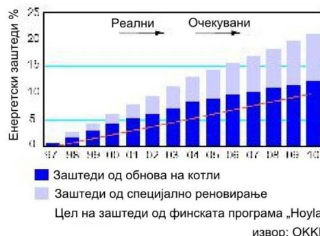
Слика 1.2.2.4. Моментални и резултати што се очекуваат во период од 10 години
