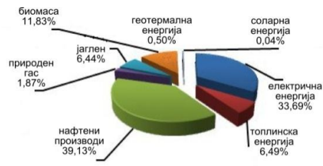
Слика 1.3. Потрошувачка на финална енергија по енергенс, во 2006 година
